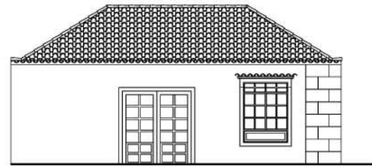
FACHADA FE01 1:150 C/ El Lomo, 4
